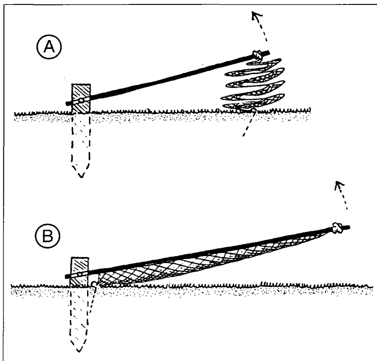
2. Dwarsdoorsneden van het opgevouwen druijnet (A) en het op de grond uitgespreide open net (B). Tekening: J. ter Pelkwijk.
